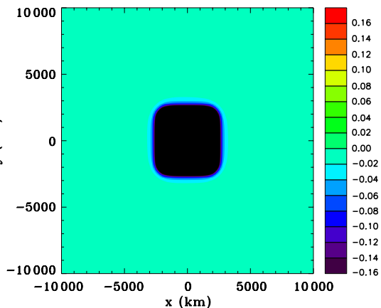
(d) Total energy perturbation
