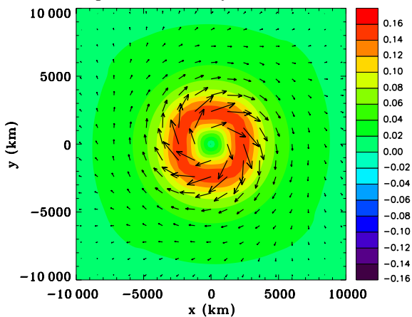
(d) Speed and velocity vectors z=15.25 km
