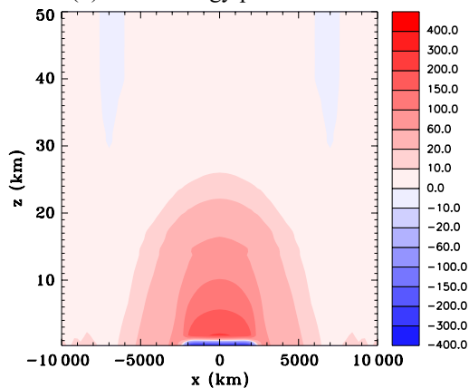
(d) Total energy perturbation
