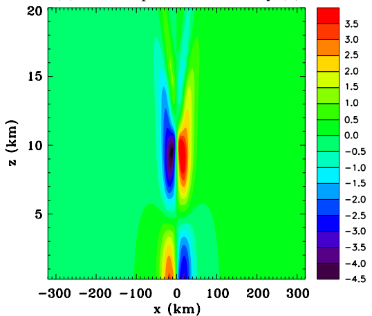
(d) x-component of velocity (u)
