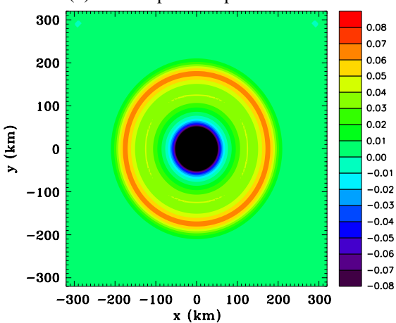
(d) Surface pressure perturbation t=10 m
