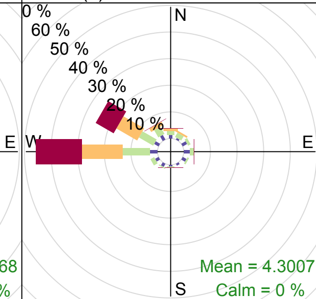
(d) RADM2-MADE/SORGAM
