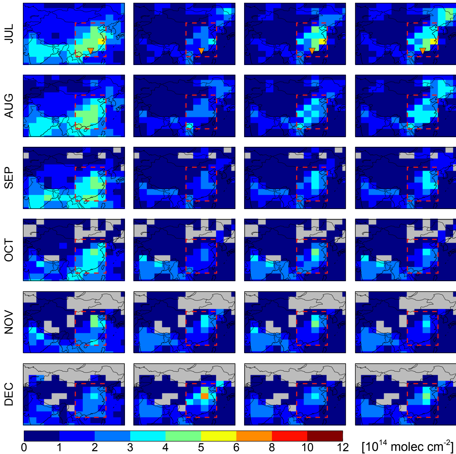
(a) GOME-2A
