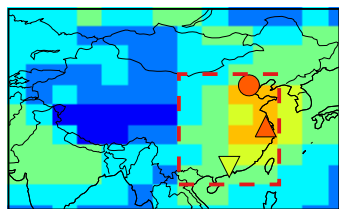
(a) GOME-2A
