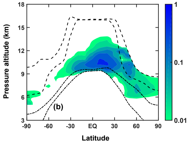
HET fraction of ice extinction
