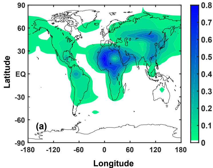
HET fraction of ice optical depth
