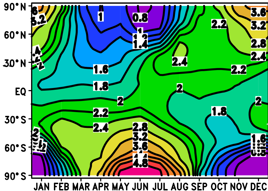
(a) WACCM-Ca Ca ( 10^7 \text{ cm}^{-2} )
