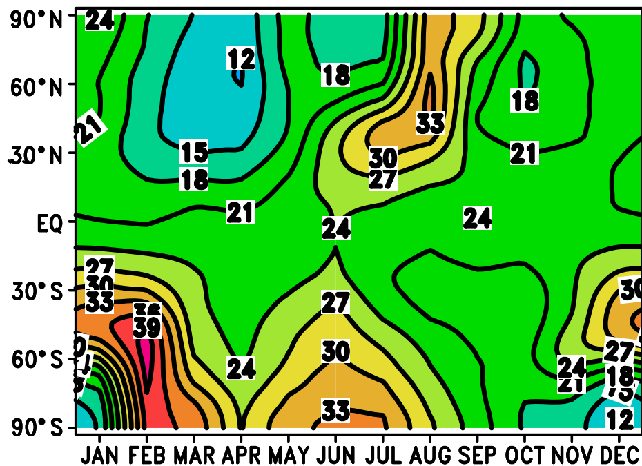
(b) WACCM-Ca Ca + ( 10^7 \text{ cm}^{-2} )
