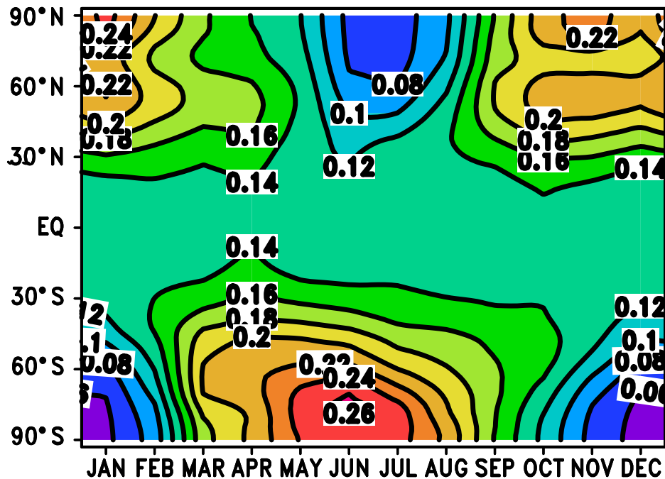
(d) WACCM Ca + /Na +
