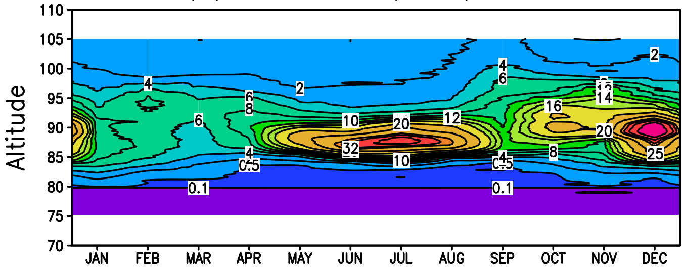
(a) Lidar Ca ( \text{cm}^{-3} ): 54° N
