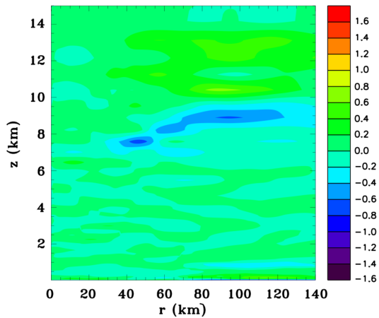
(d) Potential temperature perturbation
