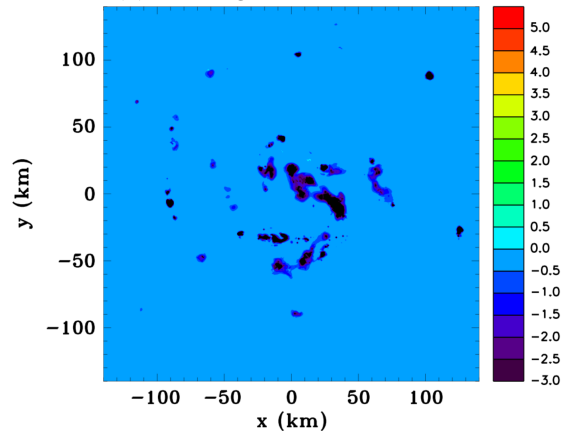
(d) Melting z = 4.3 km 48 h
