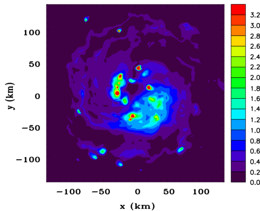
(d) Hydrometeors z = 9.5 km 60 h
