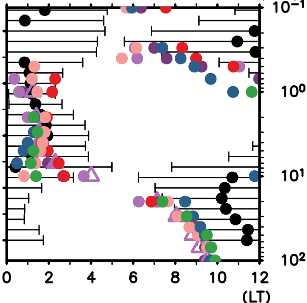
(d) Phase (30–45° N) (hPa)
