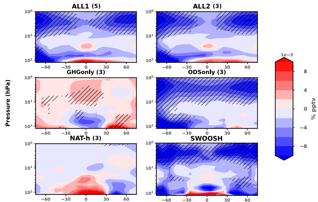
(b) Li EESC trends, 1984-2016*
