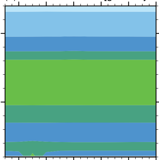
(d) AR5 BC emission [ \text{g C m}^{-2} \text{ year}^{-1} ]
