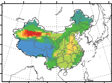
(d) MISR AOD
