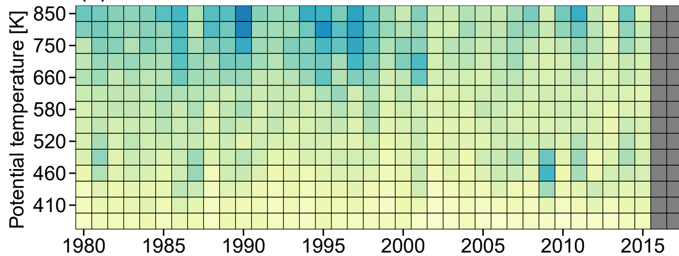
(d) ERA-I SD of diffs
