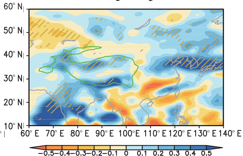
(d) Surface precipitation
