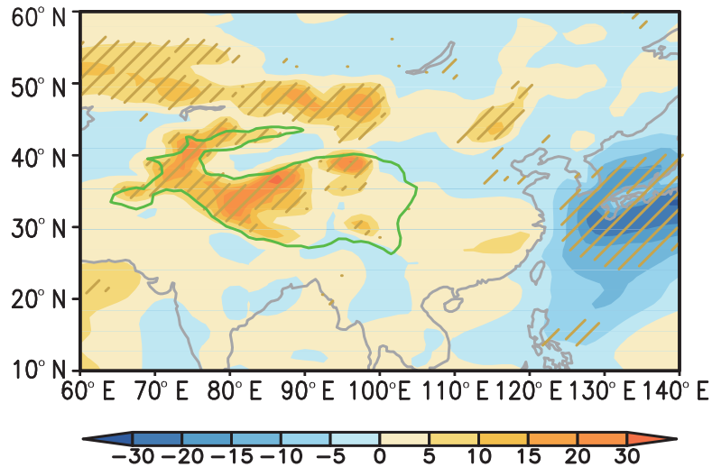
(d) Latent+sensible heat flux
