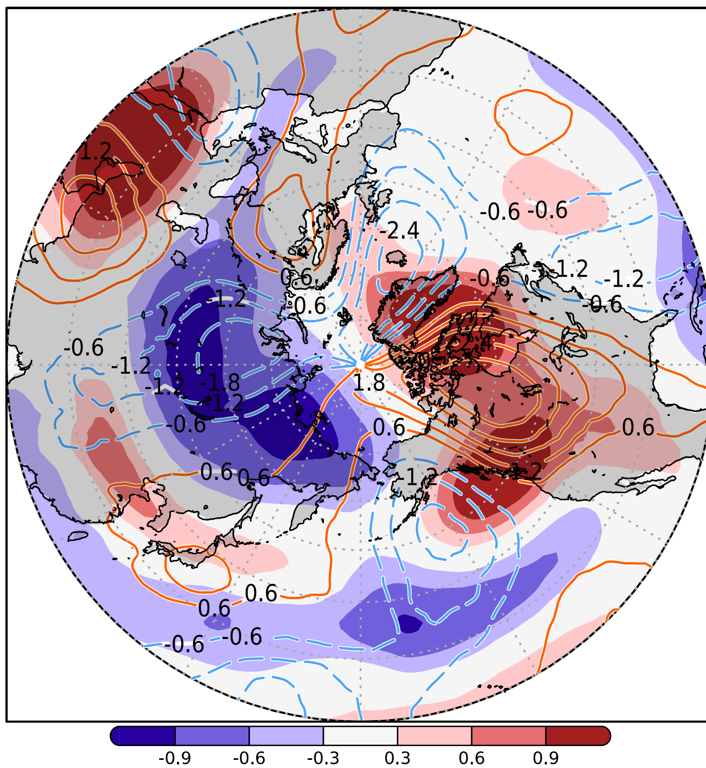
(d) Deviation of V' , T'_{100} (16NOV-30NOV)
