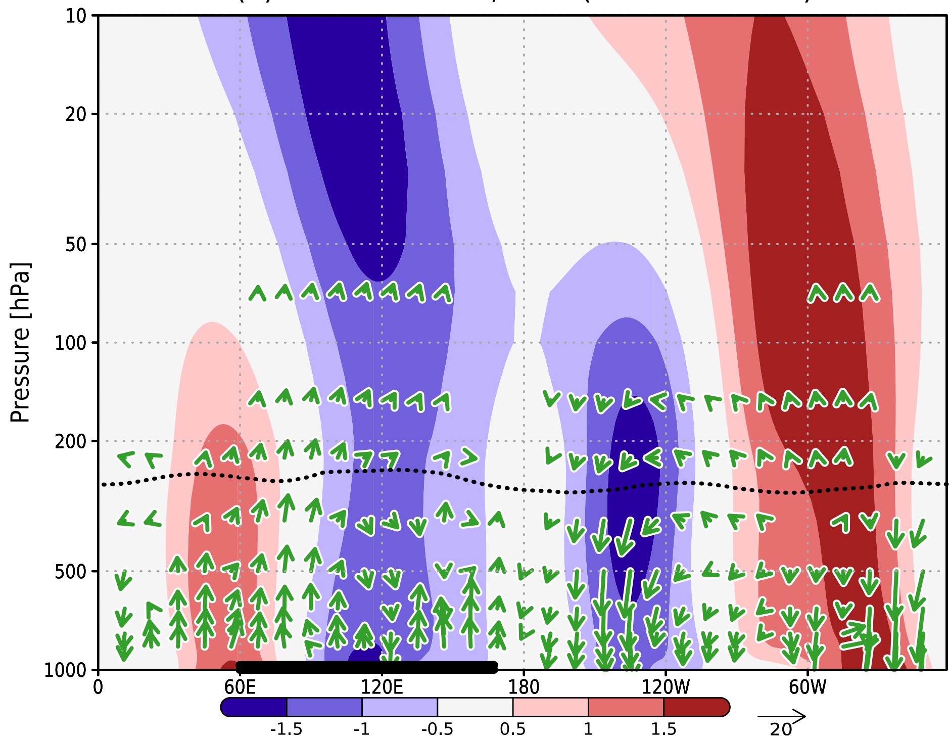
(d) Deviation of Z' , WAF (16NOV-30NOV)
