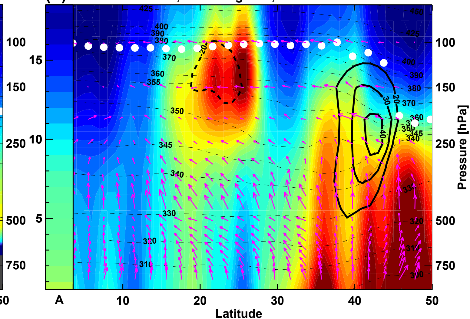
(d) IASI CO, 135.0 longitude, 2008/07/26
