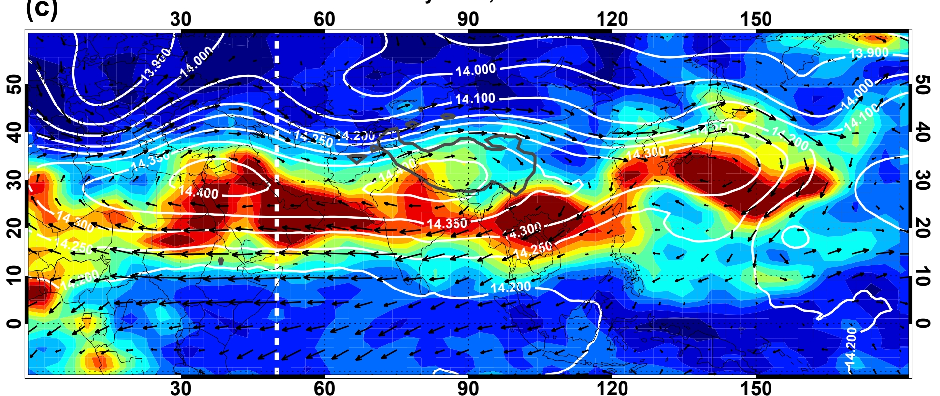
IASI UT layer CO, 2008/07/22
