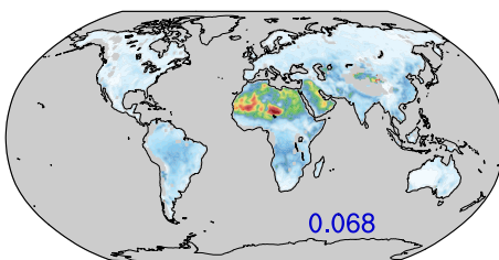
(d) SON
