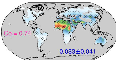
(h) SON
