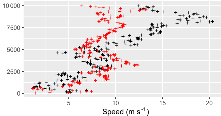
(d) Wind speed
