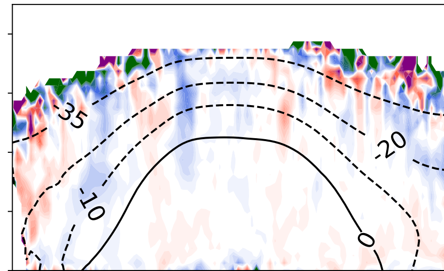
\Delta\text{LWC}
