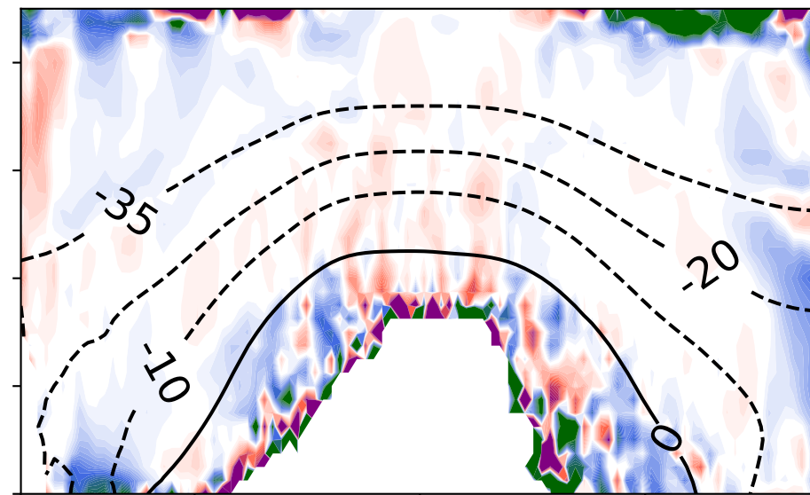
\Delta\text{IWC}
