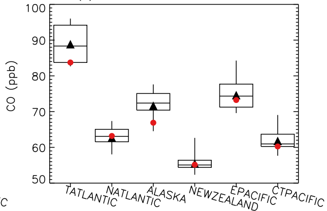
(d) MLS CO at 215 hPa
