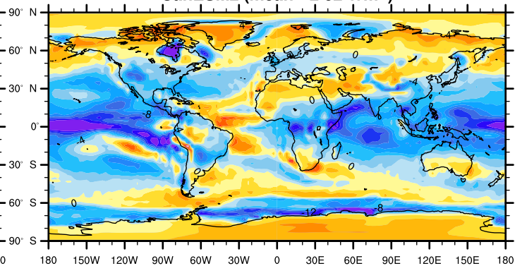
HadGEM2-ES (mean: -2.29 \text{ Wm}^{-2} )
