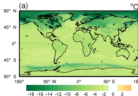
G1-abrupt4xCO2
