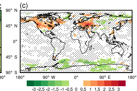
&lt;G1-abrupt4xCO2&gt;-&lt;G4-rcp45&gt;
