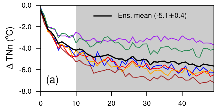
G1-abrupt4xCO2
