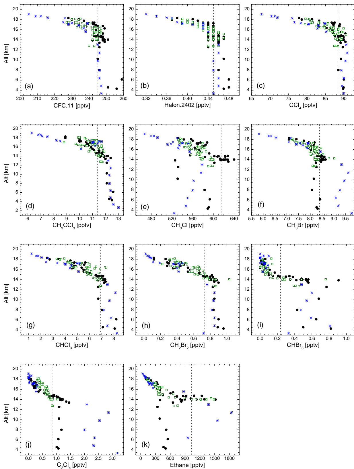
Figure S1. Vertical distributions of (a) CFC-11, (b) Halon-2402, (c) \text{CCl}_4 , (d) \text{CH}_3\text{CCl}_3 , (e)
